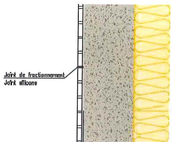
Figure 8 — Joint de fractionnement horizontal
