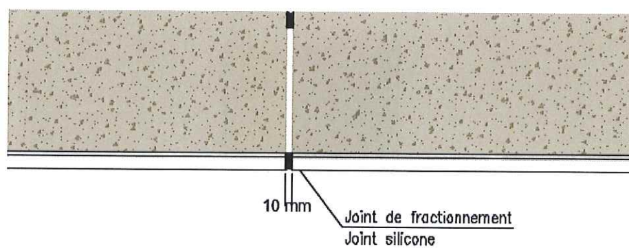
Figure 9 — Joint de fractionnement vertical
