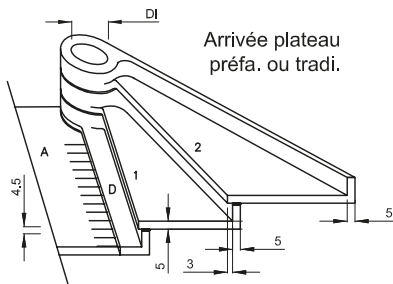
Départ encastré dans dalle finie
