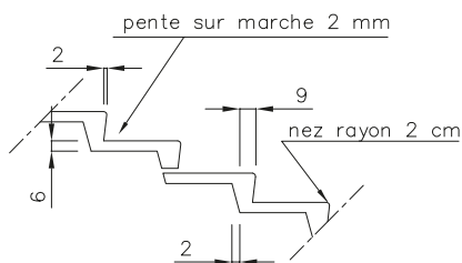
Détail sur marches
