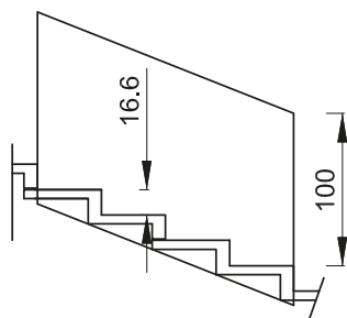
Détail sur marches
