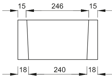
Détail du fût
