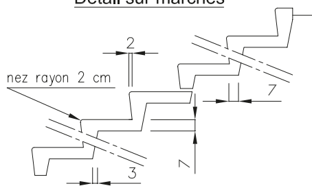
Détail sur marches
