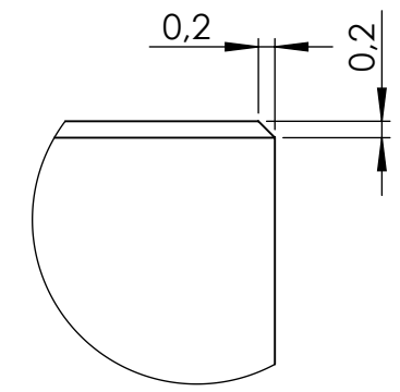
DÉTAIL F
