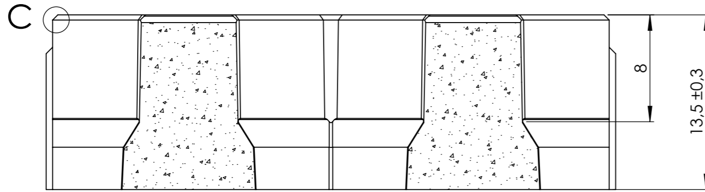
COUPE B-B
