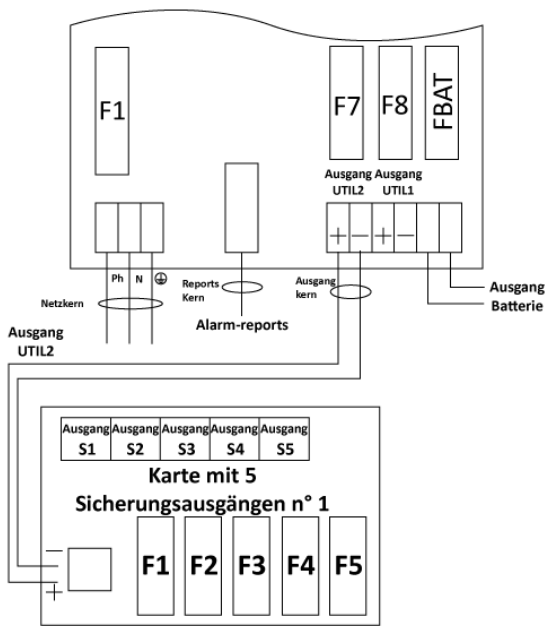
Abb. 3 Verkabelung mit der Karte mit 5 Sicherungsausgängen (serienmäßig)
