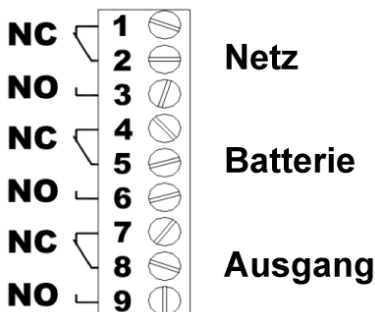
Abb. 5 Verkabelung Alarmreports
