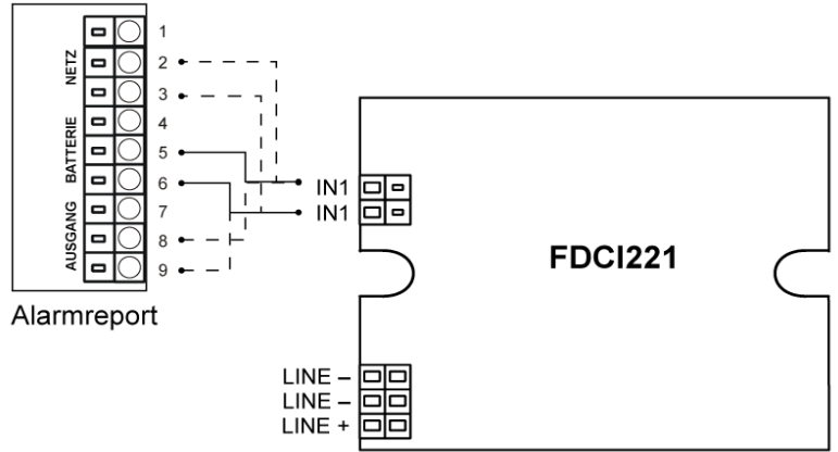
Beispiel : NO-Kontakt - Entdeckung Batteriefehler
