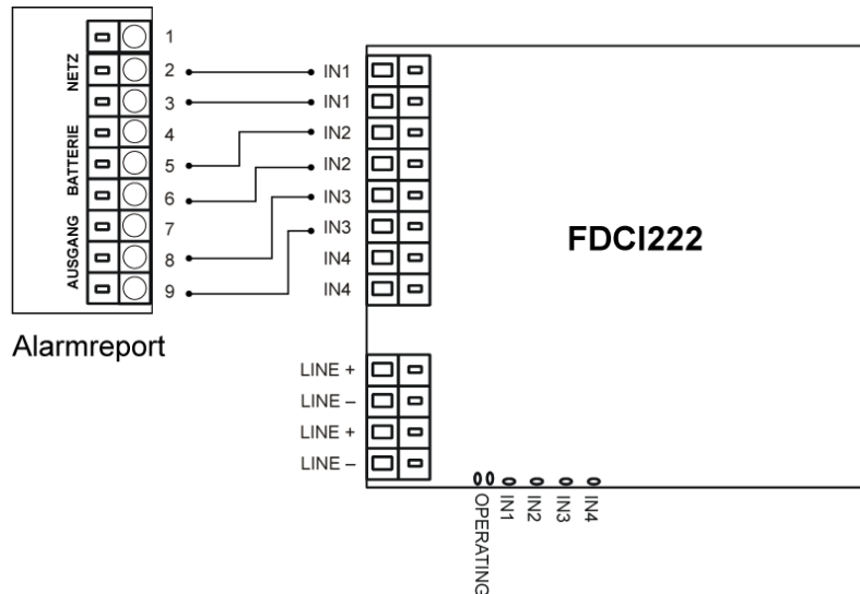
Beispiel : NO-Kontakt Entdeckung Netz-, Batterie- und Ausgangsfehler
