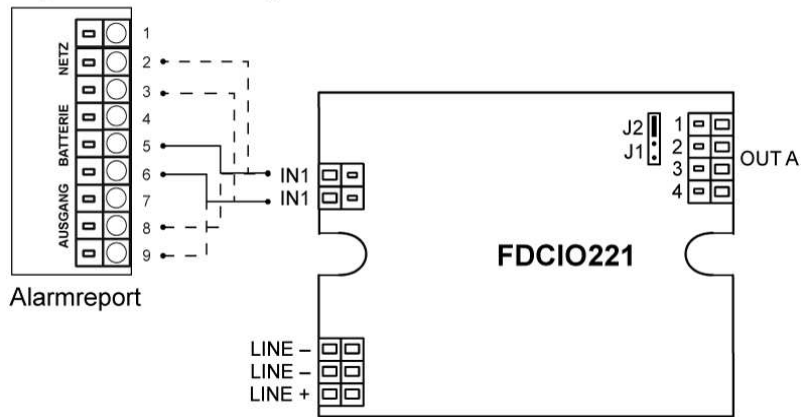
Beispiel : NO-Kontakt - Entdeckung Batteriefehler
