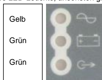
Abbildung 3: Beispiel LED-Anzeigen bei Fehler im Stromnetz
