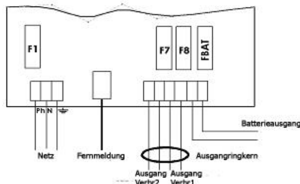
Verkabelung 100-150 W
