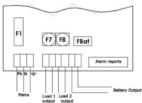
75 W wiring
