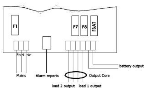
100-150 W wiring
