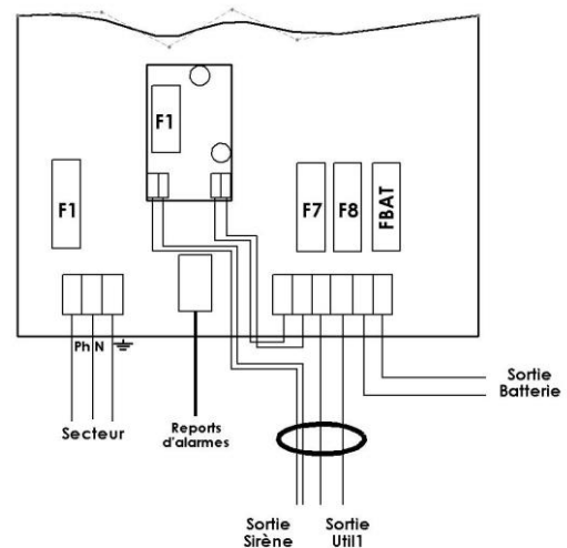
Câblage option sirène – 100 / 300W
