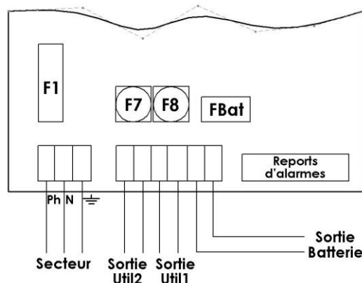
Câblage 75W
