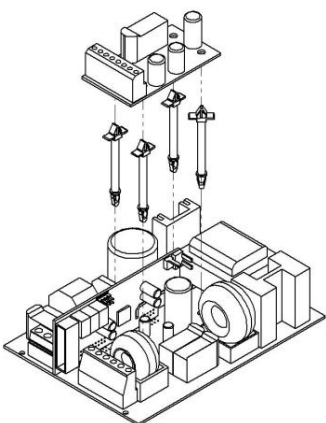
Siren option 100 - 150 W
