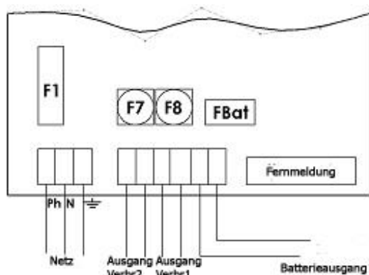
Verkabelung 75 W
