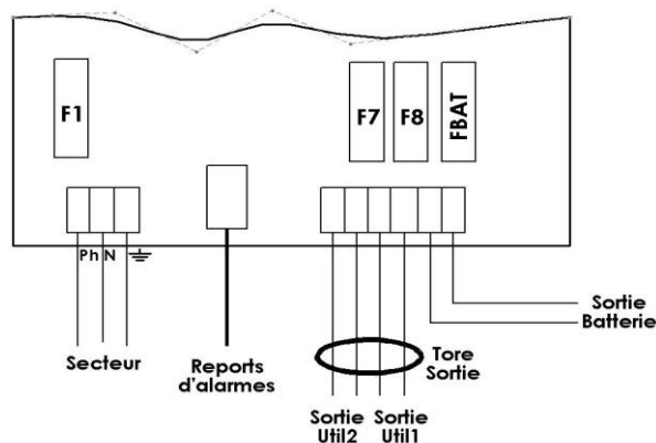
Câblage 100-150W
