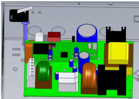
C24 schakelaar
