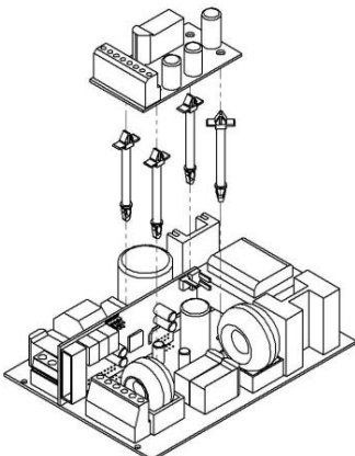
Sirene-Option 100-150 W
