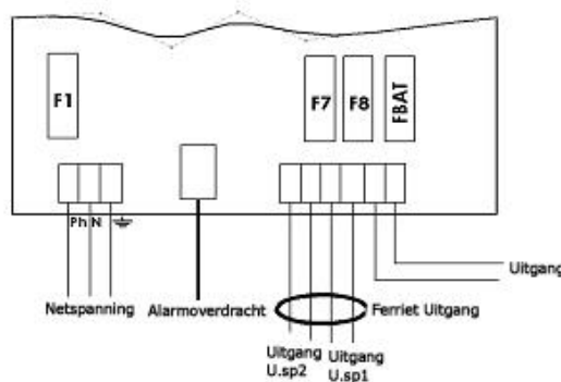
Kabels 100-150W
