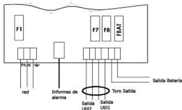
Cableado 100-150 W
