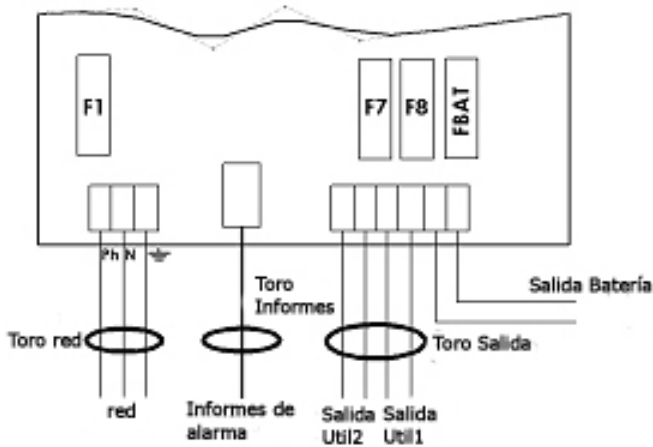
Cableado 400-600 W
