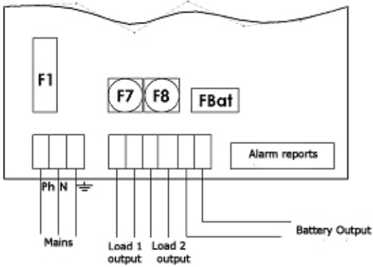
75 W wiring
