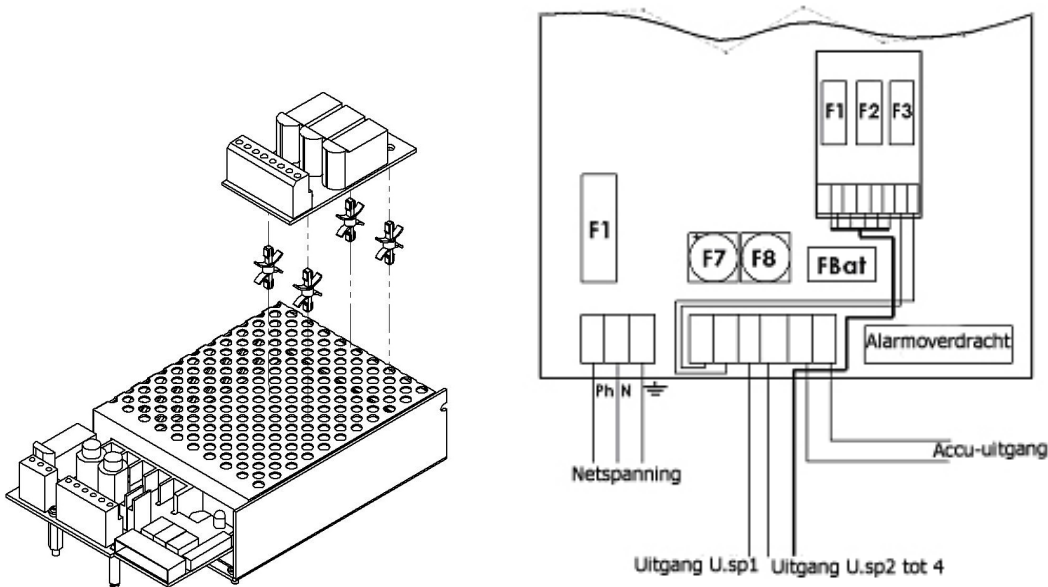
Kaart met 3 afgezekerde uitgangen - 75W
