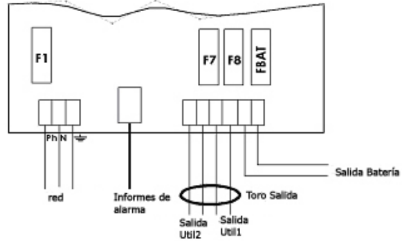
Cableado 100-300 W
