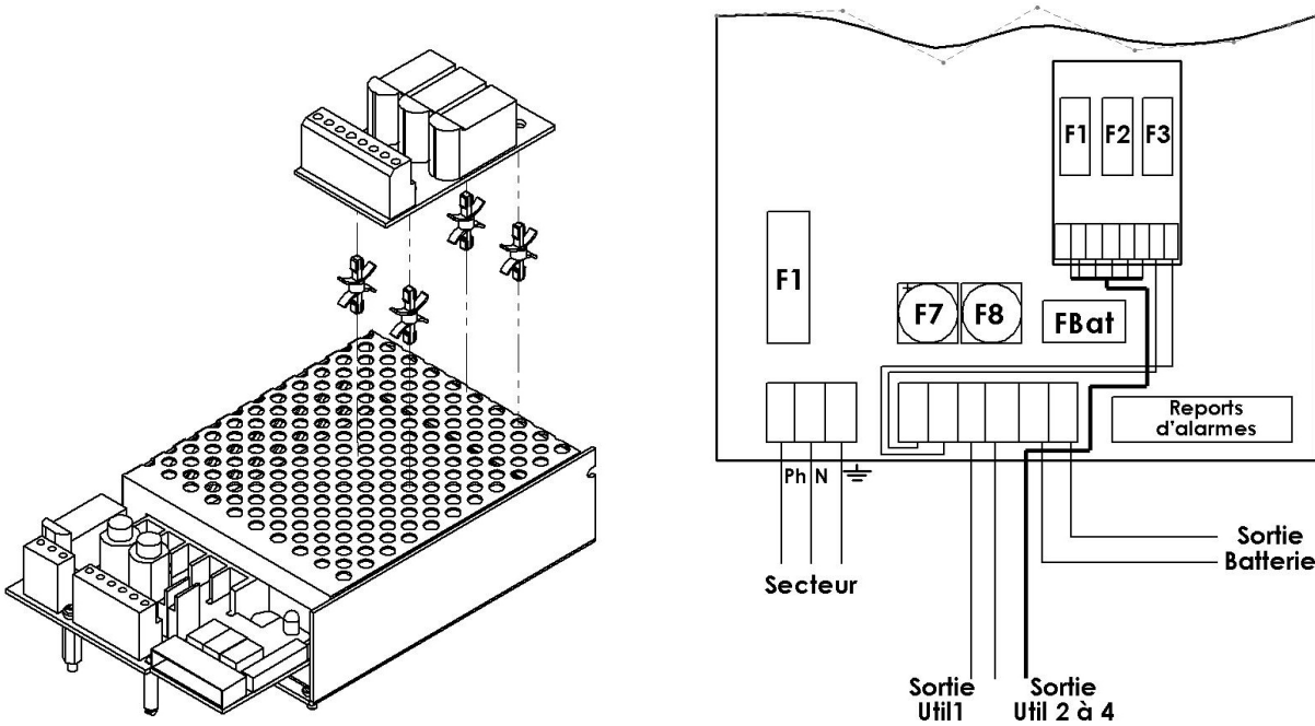
Carte 3 départs fusibles 75W
