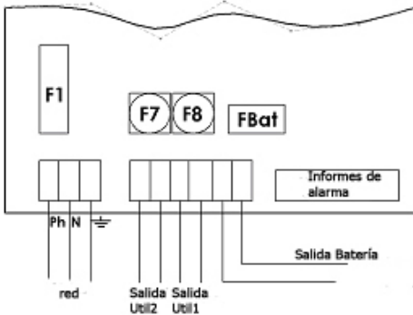
Cableado 75 W
