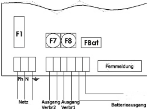
Verkabelung 75 W
