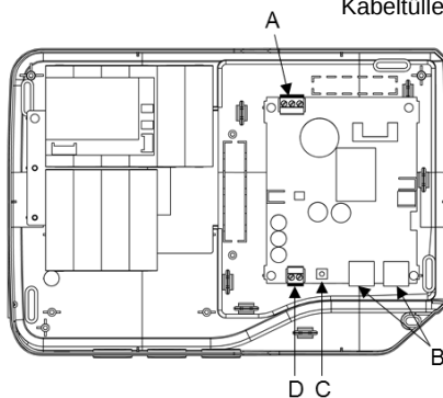
Fig. 3: BOX2 55W
